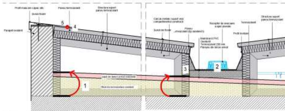
Figura 1. Schema adaptărilor propuse VARIANTA 1
