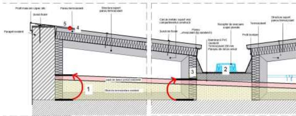
Figura 1. Schema adaptărilor propuse VARIANTA 1
