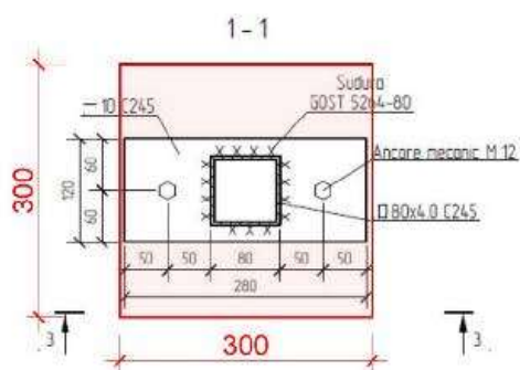
Figura 4. Nod talpă de sprijin a construcției metalice de placa de beton.
