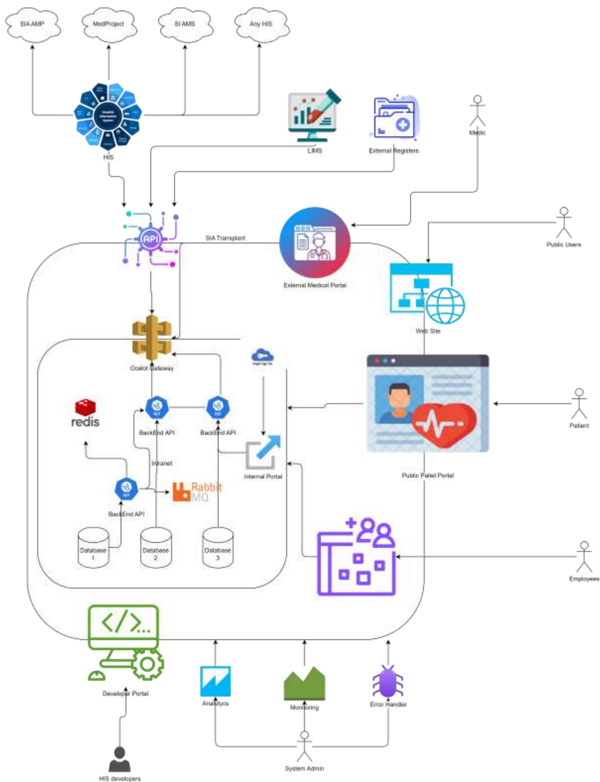
Figura 4. Arhitectura generală SI Transplant
