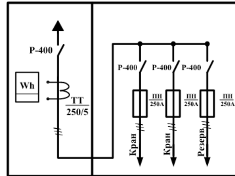
ГРЩ
