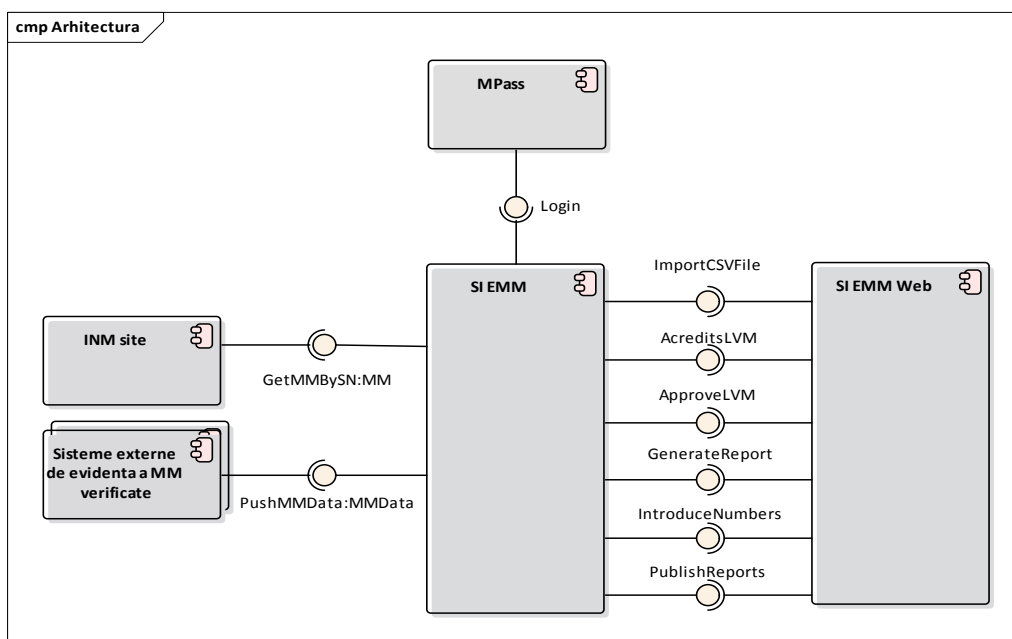
Figura 1. Arhitectura SI EMM
