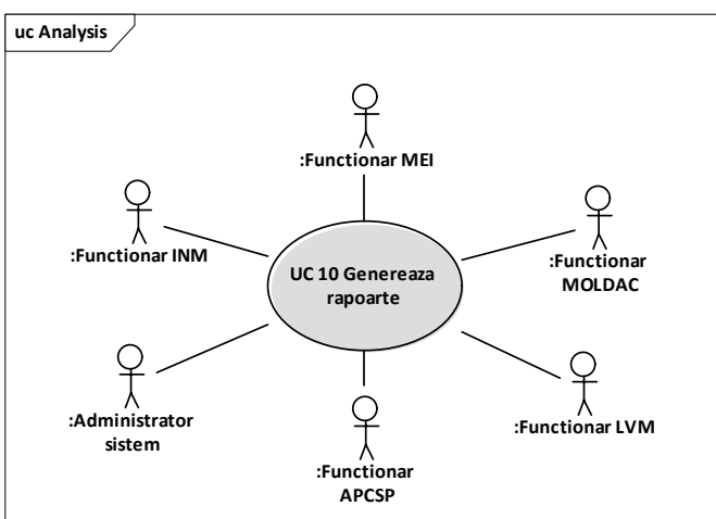
Figura 3. Funcționalitățile SI EMM
