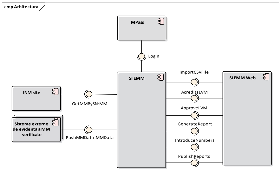
Figura 1. Arhitectura SI EMM
